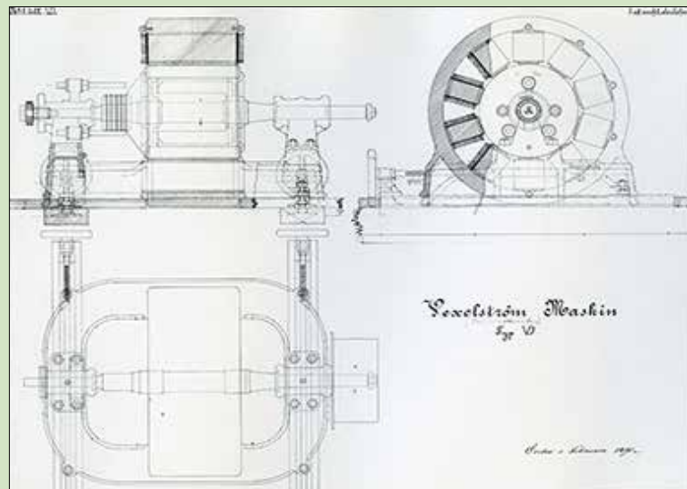
Ritning av växelströmsmaskinen
